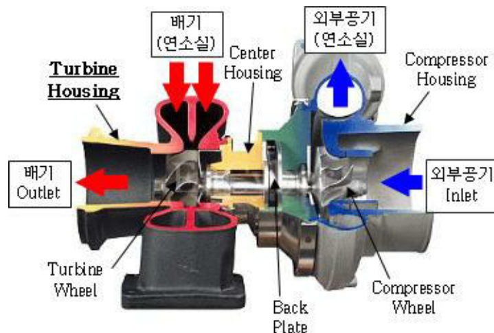
자동차 터보의 구조
