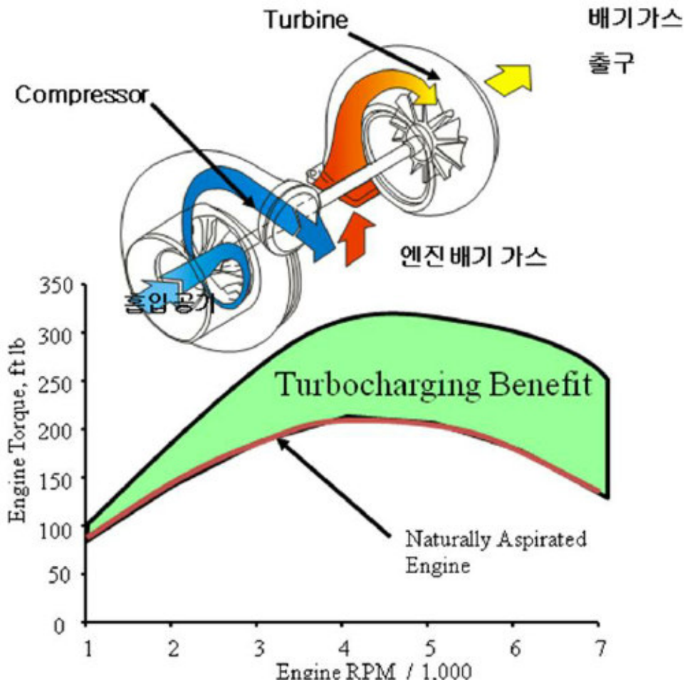
터보차저의 장점
